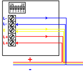
ML - 1420.SCI AKILLI ADRESLİ SİSTEM FLAŞÖR KISA DEVRE İZOLATÖRLÜ
