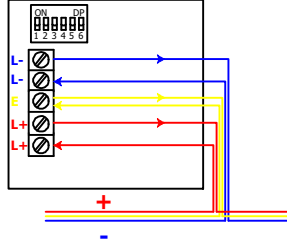
ML-1430.SCI AKILLI ADRESLİ SİSTEM FLAŞÖRLÜ SİREN KISA DEVRE İZOLATÖRLÜ
