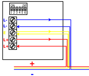
ML - 1420 AKILLI ADRESLİ SİSTEM FLAŞÖR
