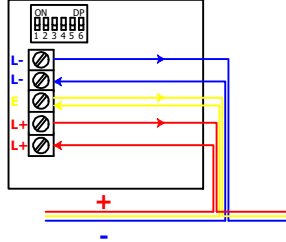
ML - 1430 AKILLI ADRESLİ SİSTEM FLAŞÖRLÜ SİREN
